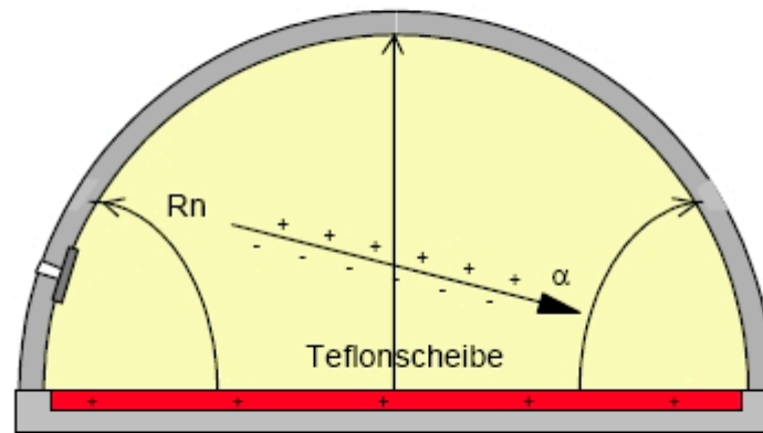
Diffusionskammer aus leitendem Kunststoff
