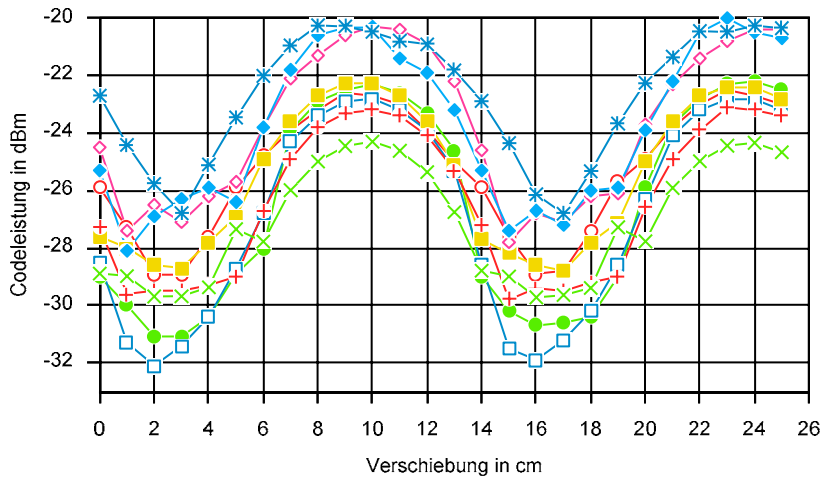
Fig. 5 Gemessene Codeleistung mit 9 verschiedenen Geräten in Funktion der Verschiebung
