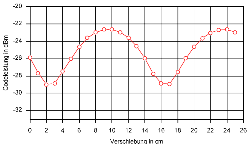
Fig. 4 Erwarteter Messwert der Codeleistung in Funktion der Verschiebung (Thermischer Leistungsmesser anstelle des zu kalibrierenden Messgerätes, korrigiert um die relative Codekanalleistung entsprechend der Generatoreinstellung)
