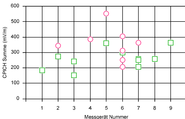
Fig 2: Vergleichsmessung auf der Terrasse
