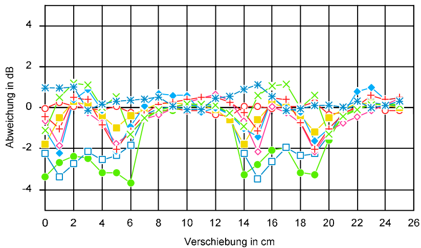
Fig. 7 Abweichung vom erwarteten Wert (Fig. 4), Messwerte korrigiert mit Korrekturfaktor
