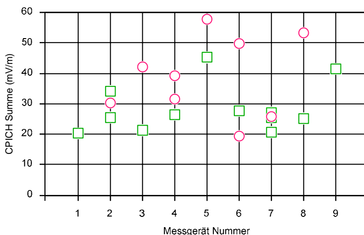
Fig. 1: Vergleichsmessung im Sitzungszimmer
