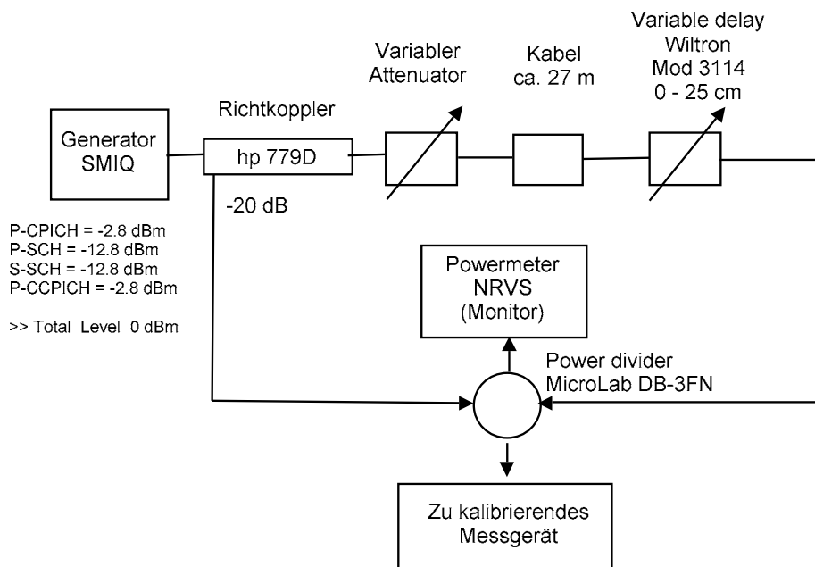
Fig. 3 Messaufbau für den Test im Labor mit Mehrwegausbreitung
