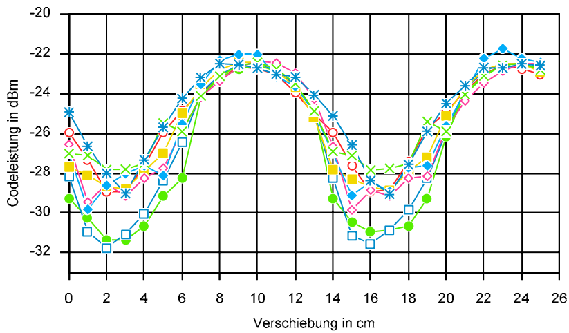
Fig. 6 Gleiche Messungen wie Fig. 5. Messwerte korrigiert mit Korrekturfaktor
